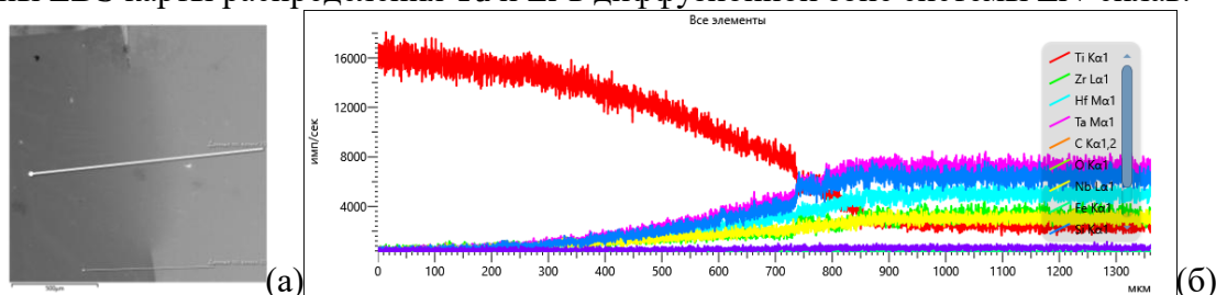
Рисунок 1. Типичная зона сварного соединения (а) системы Ti / сплав после отжига по режиму А (фотография SEM); зависимость интенсивности отраженного излучения от глубины проникновения элементов сплава (б)
