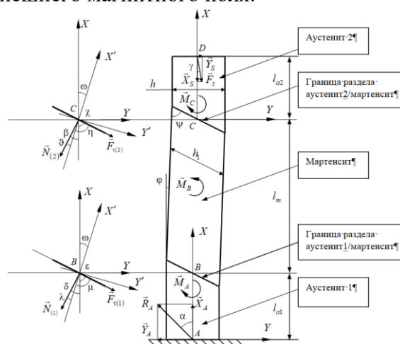
Схематическое изображение сжимаемого пружиной исполнительного элемента Ni_2MnGa , используемого в электромагнитном приводе
