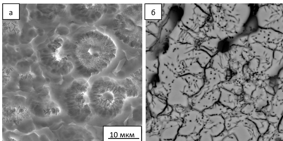
Рис.1. – структура сплава Ni-Co-Si-Ti-Al до(а) и после (б) отжига.
