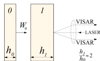
Рис.1. 0 – ударник со скоростью W_0 \approx \text{const} , 1- образец.
