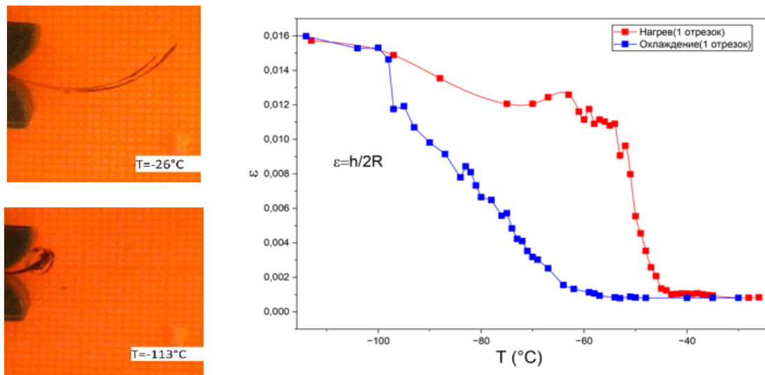
Рис. 1. Двусторонний ЭПФ в быстрозакаленной ленте ферромагнитного сплава Гейслера из переходных 3d элементов Ni 37 Co 13 Mn 35 Ti 15 . (а) образец ленты сплава в аустенитной высокотемпературной фазе. (б) образец в мартенситной низкотемпературной фазе. (в) график зависимости изгибной деформации образца от температуры.
