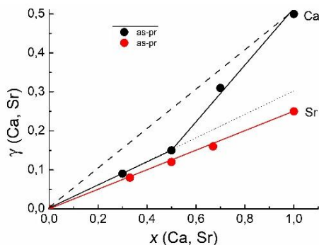
Рис.3. Зависимость числа кислородных вакансий от количества ионов Ca, Sr.
