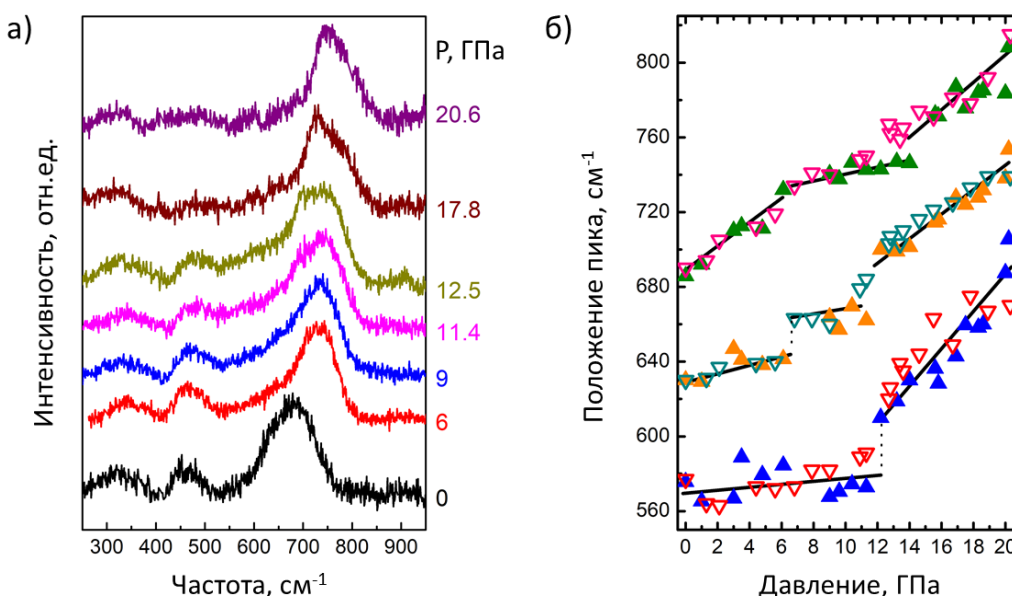
Рис. 1 а) спектры КРС образца \text{La}_{0.5}\text{Sr}_{0.5}\text{FeO}_{2.75} при повышении давления (величины давлений в ГПа даны справа); б) зависимости положений мод, соответствующих колебаниям октаэдра \text{FeO}_6 , при повышении (закрытые символы) и понижении (открытые символы) давления.
