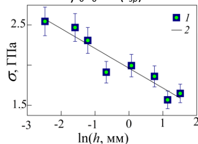
Рис.3. Линейная зависимость откольной прочности \sigma от логарифма толщины откольной пластины \ln(h) .
