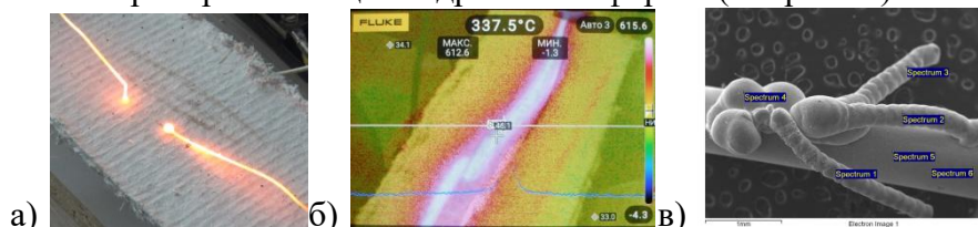
Рисунок 1. Результаты эксперимента, а-разрушение проводника, б-максимальная температура проводника в момент разрушения, в-точки микроанализа, увеличение 35\times .
