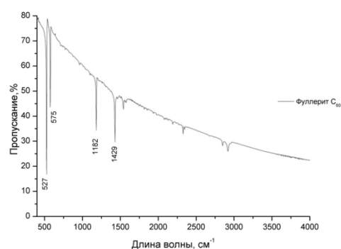
Рис. 2. ИК спектр монокристалла фуллерита
