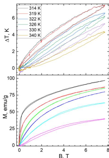
Рис.1. МКЭ в \text{Mn}_{0.93}\text{Ti}_{0.07}\text{As} , измеренный прямым методом в импульсном магнитном поле 7,6 Тл.
