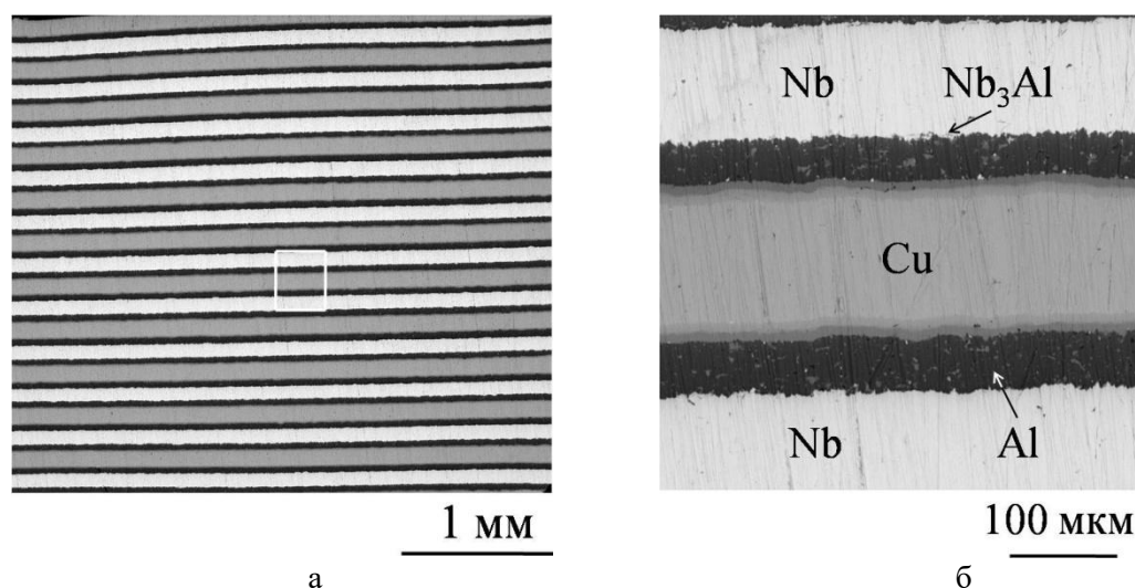
Рис. 1. Структура участка образца в поперечном сечении: а – рамкой выделена область, показанная на рис. 1б; б – участок, выделенный на рис. 1а.
