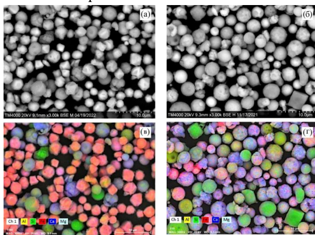
Рисунок 1 – СЭМ-снимки и карты распределения элементов магнитной (а, в) и немагнитной (б, г) фракций дисперсных микросфер золы-уноса
