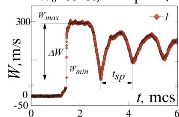
Рис.2. Скорость свободной поверхности W(t) и определение \sigma = 0.5 \rho_0 C_0 \Delta W(t_{sp})
