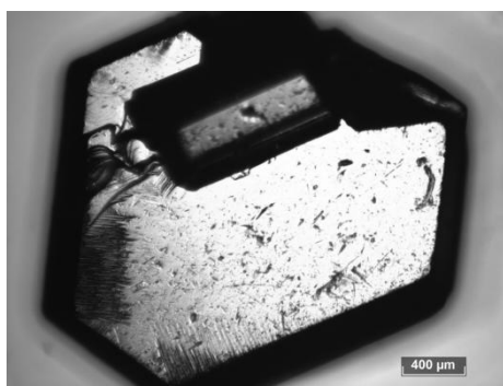
Рис. 1. Монокристалл фуллерита
