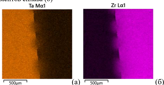
Рисунок 2. Диффузионная зона системы Zr / сплав после отжига по режиму А; фотографии EDS карт распределения Ta [элемент сплава] (а) и Zr [элемент диффузионной пары] (б)
