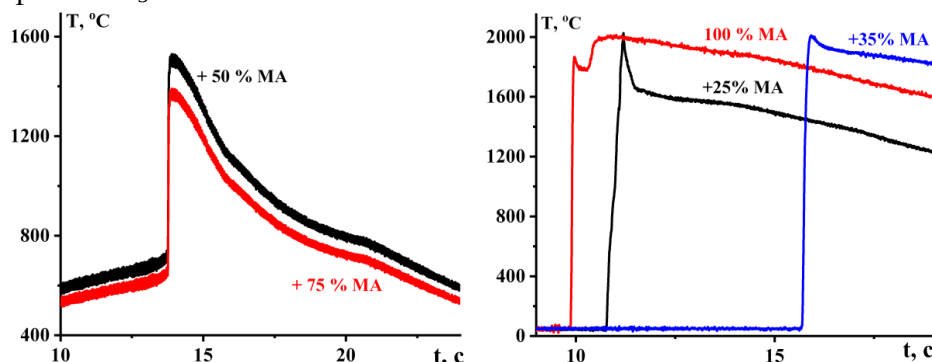
Типичные термограммы волн горения Ti-2Al-Nb и 3Nb_2O_5-6Ti-10Al в среде аргона при давлении 10^5 Па.
