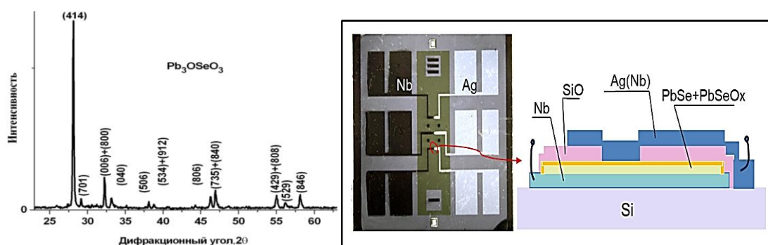
Рис.1. а) - дифрактограмма пленки PbSe, отожженной при T=500^{\circ}\text{C} в течение 3-х часов. б) - схема трех переходов Ag/ PbSeOx /PbSe/Nb, полученных фотолитографическим методом.
