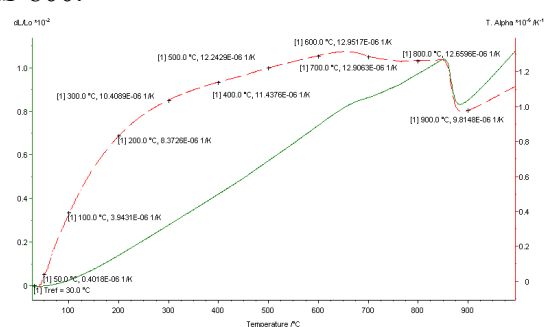
Рис.2. Изменение ТКЛР и относительных размеров образца при скорости нагрева 15 °С /мин
