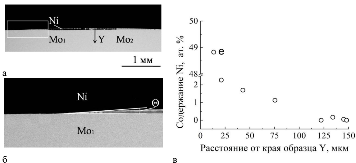
Рис. 1. Участок вертикального сечения образца (а): \text{Mo}_1 и \text{Mo}_2 – монокристаллы молибдена с вертикальной межзеренной границей (темного цвета), Ni – область, содержащая никель, Y – ось вдоль межзеренной границы, рамкой выделена область, показанная на рис. 1б; б – область, выделенная на рис. 1а, \theta – угол смачивания; в – зависимость содержания никеля по межзеренной границе от верхней кромки образца вдоль оси Y, показанных на рис. 1а, «точка» «е» в поле графика – содержания никеля в области эвтектики у верхней поверхности образца.
