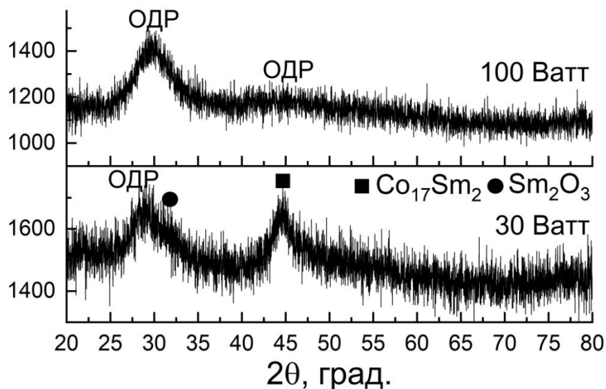
Рис. 1. Дифрактограммы Co-Sm покрытий, сформированных на Si-подложке при различных мощностях, подаваемой на Sm мишень. Здесь, ОДР – область диффузного рассеяния
