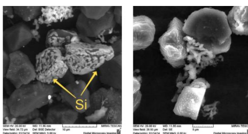
Рис. 1. Частицы алмаза АСМ 14/10 с кремниевым покрытием (а) и дендритные агломераты кремния между зернами (б)
