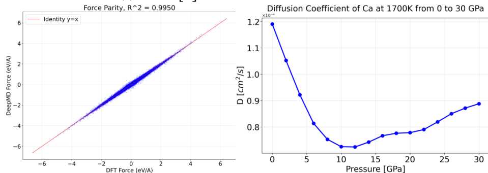
Рис. 1. (слева) Сопоставление компонент атомных сил, рассчитанных в DFT и DPA-2; (справа) Зависимость коэффициента самодиффузии жидкого Ca от давления при T = 1700 К.
