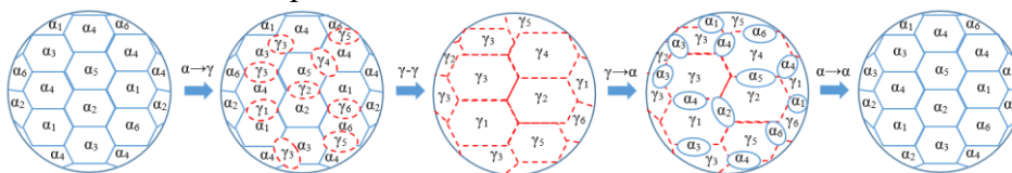
Рисунок 1. Схематическое изображение механизма текстурной наследственности при \alpha_{\text{ОЦК}} \rightarrow \gamma_{\text{ГЦК}} \rightarrow \alpha_{\text{ОЦК}} превращениях в IF-сталях
