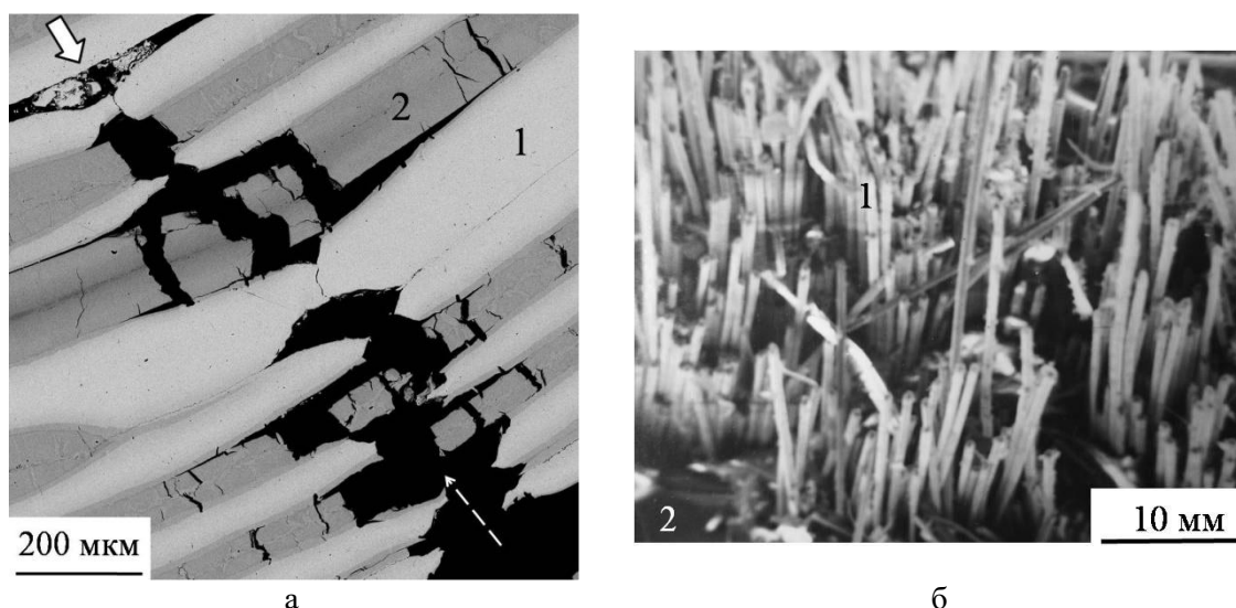
Рис. 1. Участок продольного сечения образца Ni/Al слоистого композита после испытания на трехточечный изгиб с макротрещиной: 1 – слои твердого раствора алюминия в никеле, 2 – слои Ni-Al интерметаллидов ( \text{Ni}_3\text{Al} , \text{NiAl} , \text{Ni}_5\text{Al}_3 ), сплошная стрелка – направление приложения нагрузки, пунктирная – направление распространения макротрещины (а); б – участок поверхности разрушения волокнистого углепластика после испытания на растяжение: 1 – пучки углеволокон, 2 – эпоксидная матрица.
