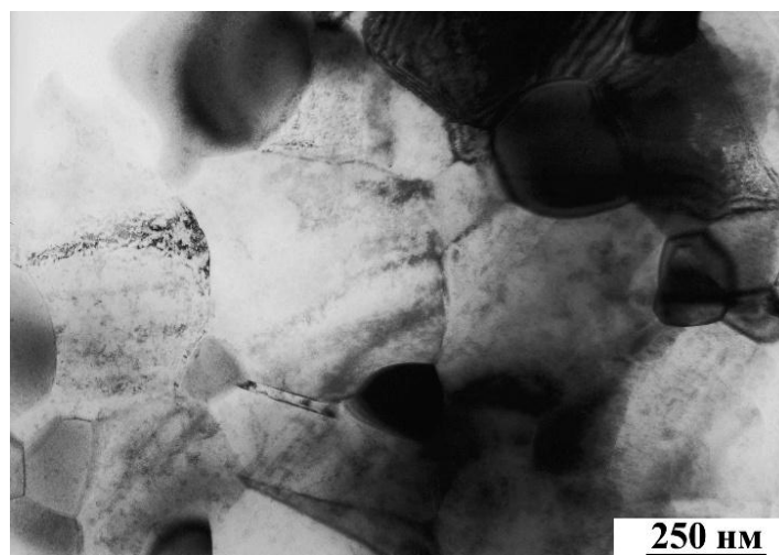
Рис. 1. Микроструктура аморфного сплава после отжига при 950 °С.
