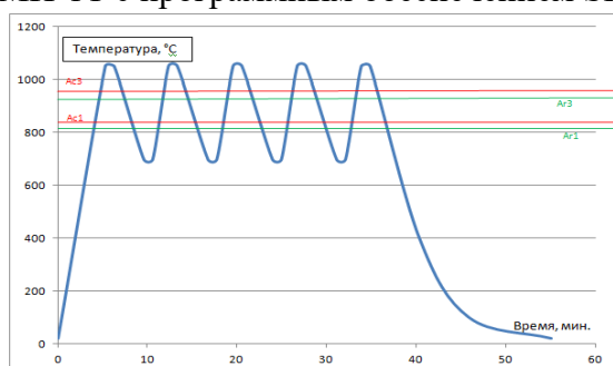
Рис.1. Высокотемпературное пятикратное термоциклирование 1050 – 700 °С
