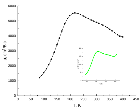
Рис.1 Температурная зависимость подвижности носителей заряда \mu ; вставка: удельная электропроводность.
