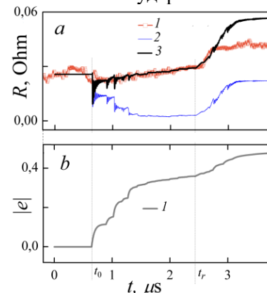
Рис.2. Профили электросопротивления (а) и интеграла абсолютной величины скорости деформации (б).
