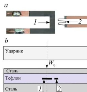
Рис.1. а – измерительная ячейка; б- генератор ступенчато-циклического нагружения; 1- вольфрамовый образец, 2- манганиновый датчик давления; W_0 = 1.05 км/с - скорость алюминиевого ударника.
