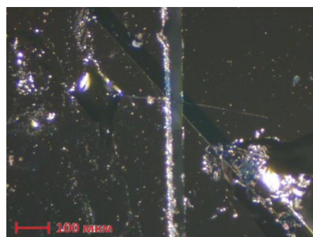
Рис. 2. Подвешенный вискер \text{TaS}_3 .
