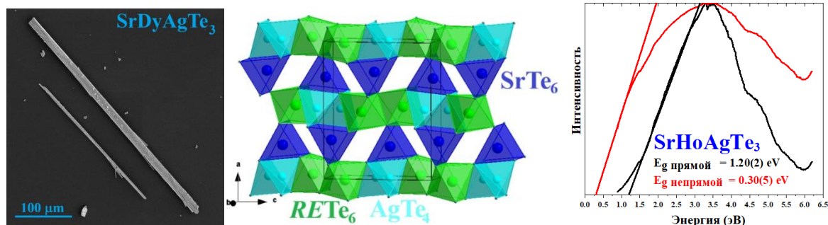
Рисунок 1. РЭМ изображение кристаллов (слева), кристаллическая структура изоструктурных соединений с общей формулой \text{SrREAgTe}_3 (в центре) и нормализованные (Кубелки–Мунка \times Энергия) a ( a = 2 , черный; 1/2 , красный) спектры \text{SrHoAgTe}_3 (справа)
