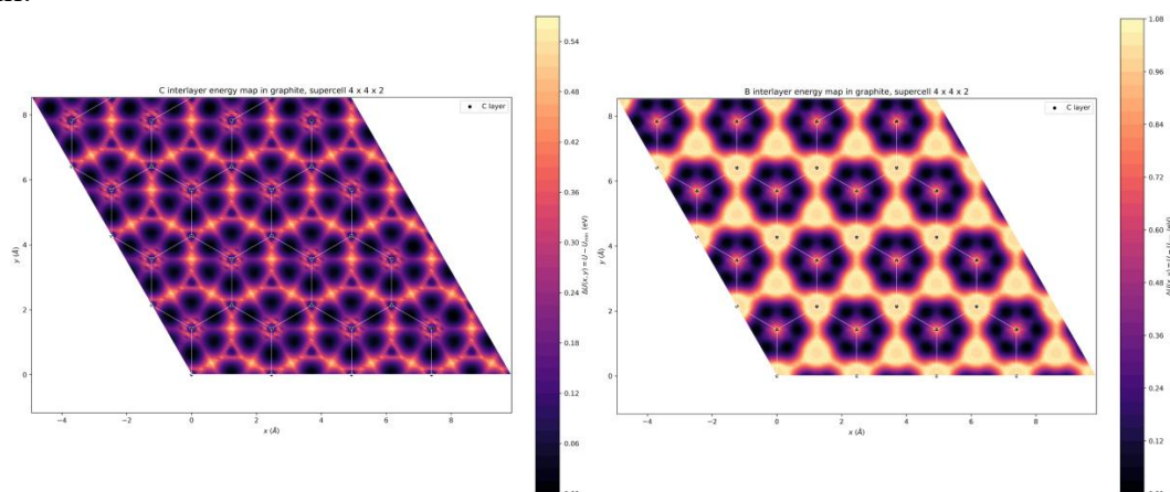
Рис. 1. Карты относительной потенциальной энергии одиночного атома С (слева) и В (справа) в межслоевом пространстве АВ-графита (сверхъячейка 4 \times 4 \times 2 ).
