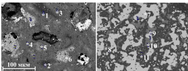
Микроструктура продуктов Ti-2Al-Nb + 75\%MA и 3Nb_2O_5-6Ti-10Al + 75\%MA
