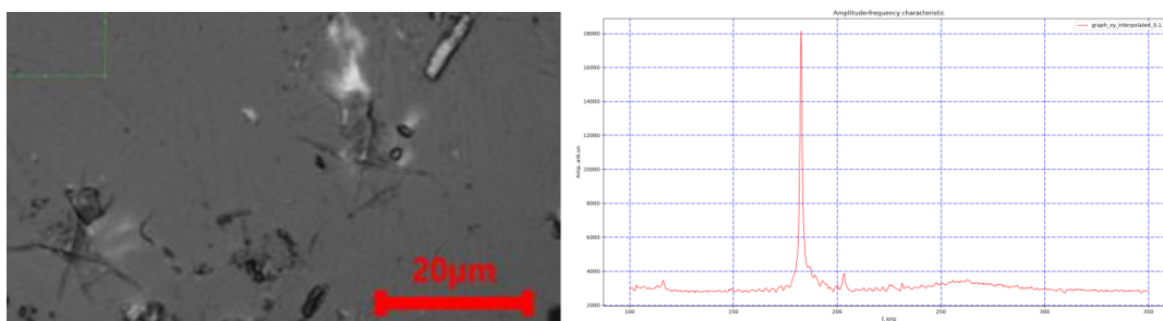
Рис.1. микротвердость по Виккерсу и УРС спектры (справа) чароита
