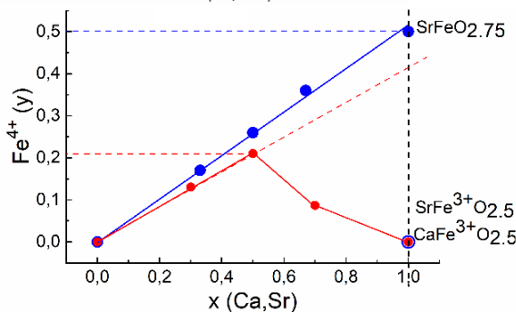
Рис.2. Зависимость количества ионов \text{Fe}^{4+} от концентрации ионов Ca, Sr.
