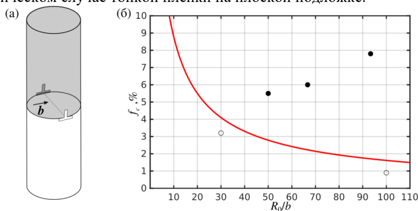
Рис. 1. а) Участок СНП с границей в частично релаксированном состоянии с дислокацией несоответствия с вектором Бюргерса b . б) Значения f_c в зависимости от радиуса СНП R_0 . Круги соответствуют реальным СНП: без дислокаций (белые), с дислокациями (черные).
