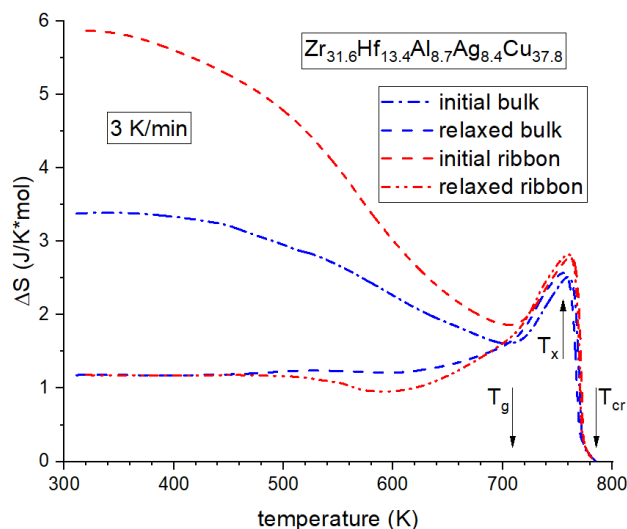
Рис. Температурные зависимости избыточной энтропии ленточных и объемных образцов МС в исходном состоянии и после релаксации.
