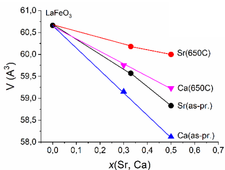
Рис.1. Зависимость объема кристаллической ячейки от количества замещающего элемента (Ca или Sr) для двух систем ферритов лантана.
