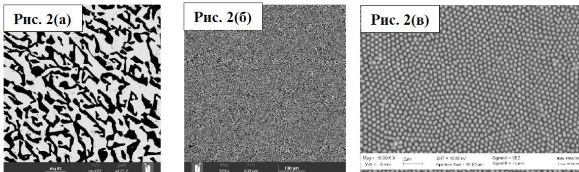
Рис. 2. Микроструктура эвтектик \text{Al}_2\text{O}_3 - \text{Er}_3\text{Al}_5\text{O}_{12} , выращенных методом EFG при скорости 10 мм/час (а) и 150 мм/час (б) и \text{Al}_2\text{O}_3 - \text{GdAlO}_3 (в)
