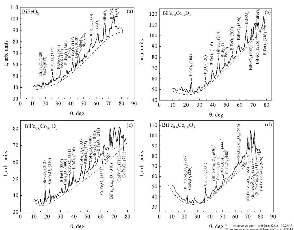
Рис. 1. Дифракционные картины от образцов \text{BiFe}_{1-x}\text{Co}_x\text{O}_3 при x=0 (a); 0,2(b); 0,4(c); 0,6(d)
